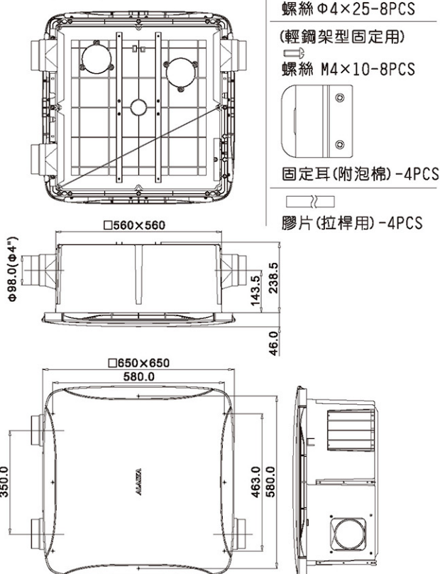
主機
