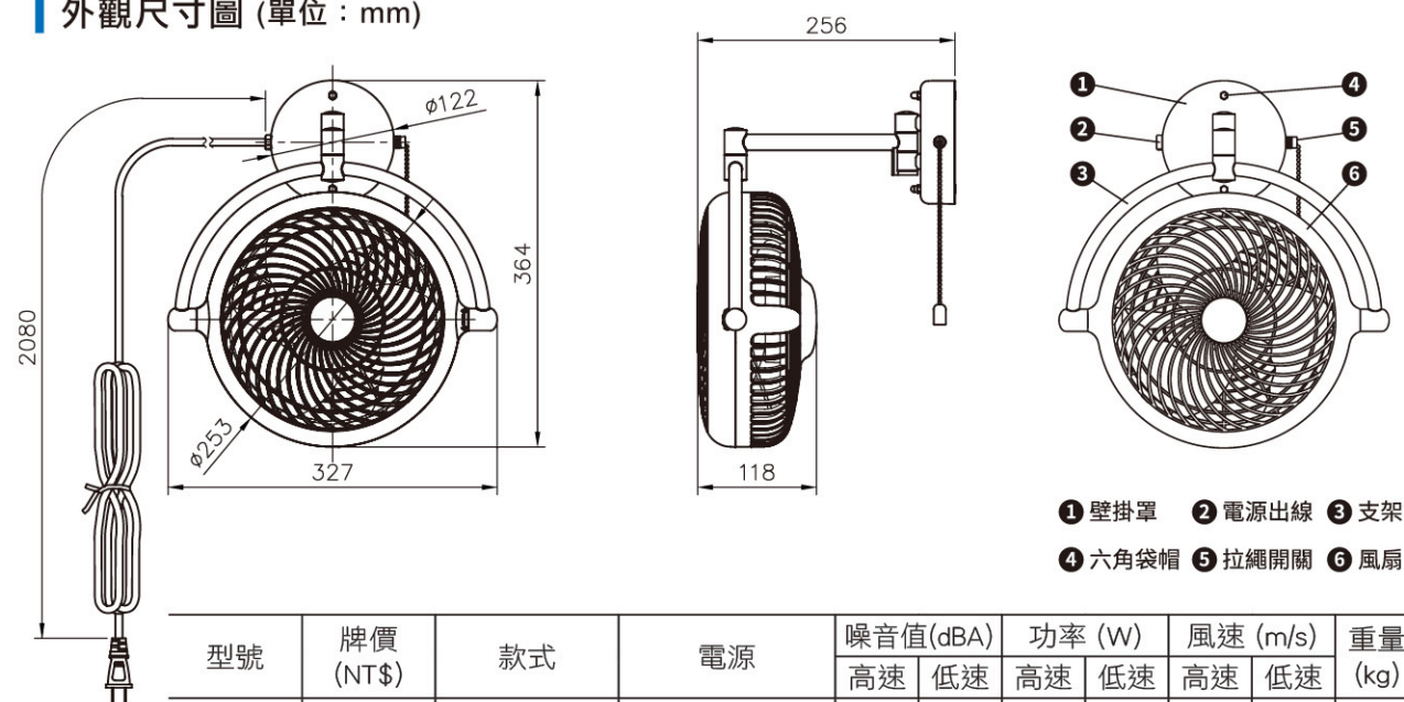
外觀尺寸圖 (單位：mm)
