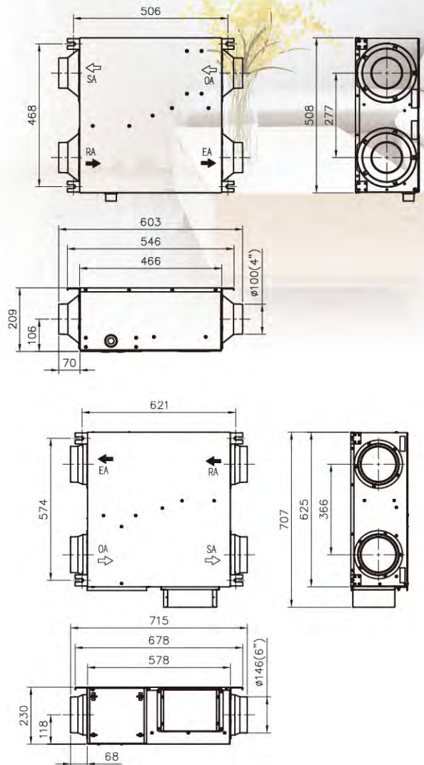
●外觀尺寸圖 (單位：mm)
